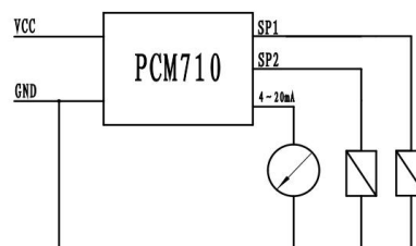
PNP 输出接线图
