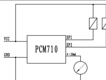
NPN 输出接线图
