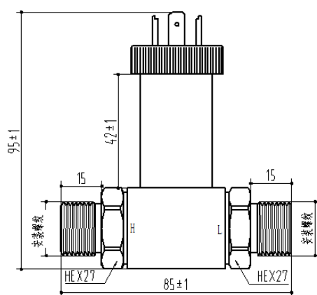
外形尺寸
